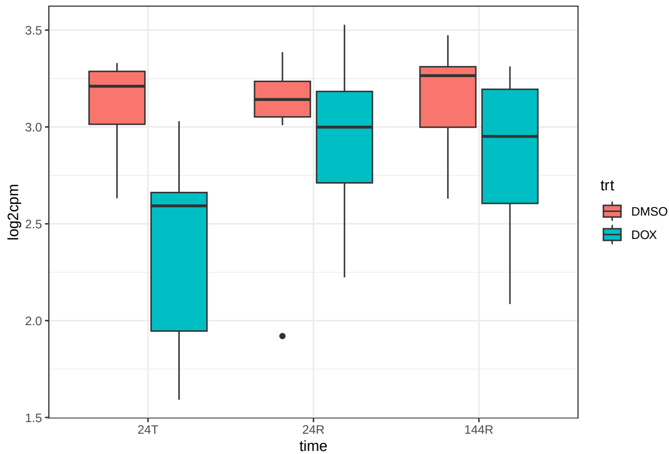
gene 339500 ZNF678
